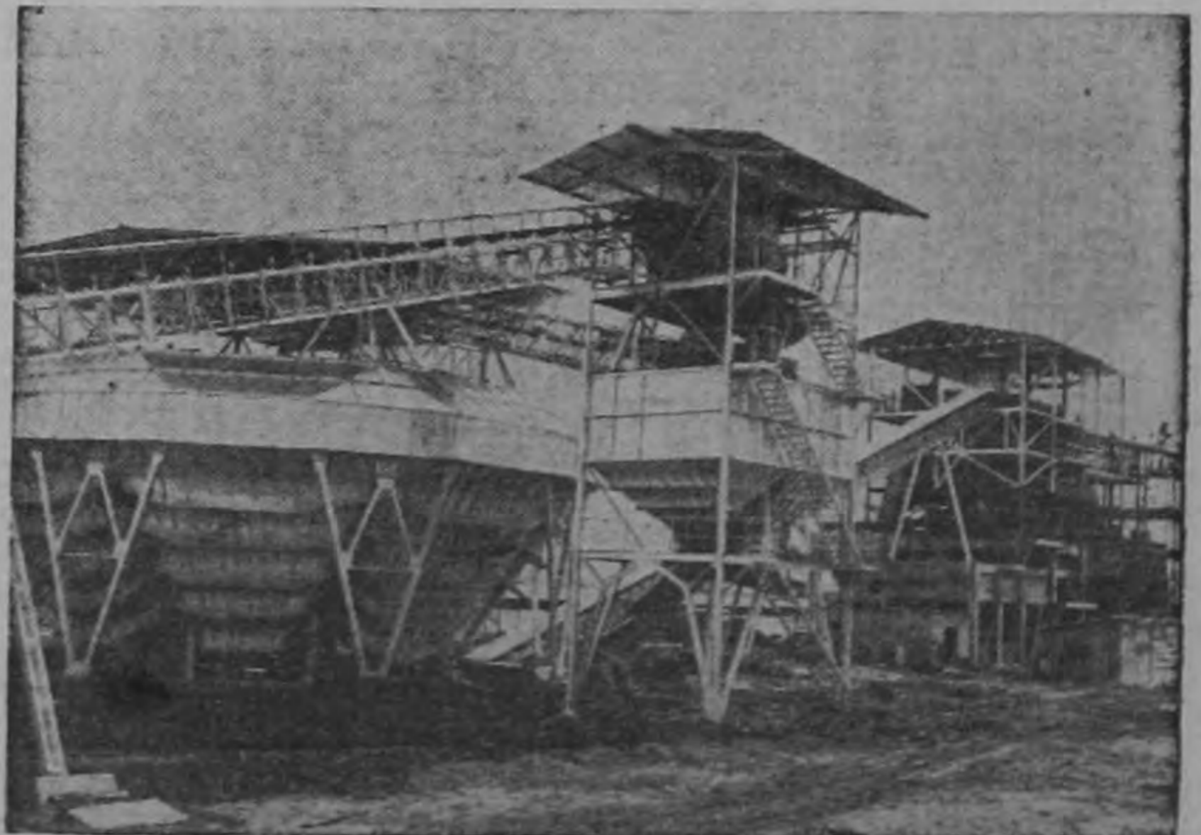
Este transbordador de correa, en una instalación para lavar carbón coke, cerca de Cali, Colombia, transporta el carbón en una de las mayores minas de la América Latina. El carbón coke indispensable para hacer acero, es uno de los productos de mayor utilidad y más escaso en Sud América. (International)
